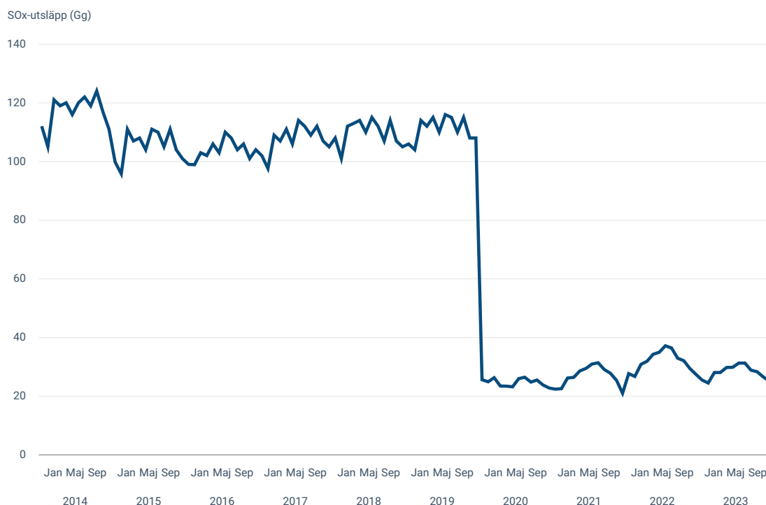
Figur 4 SOx-utsläpp för EU, 2014–2023
