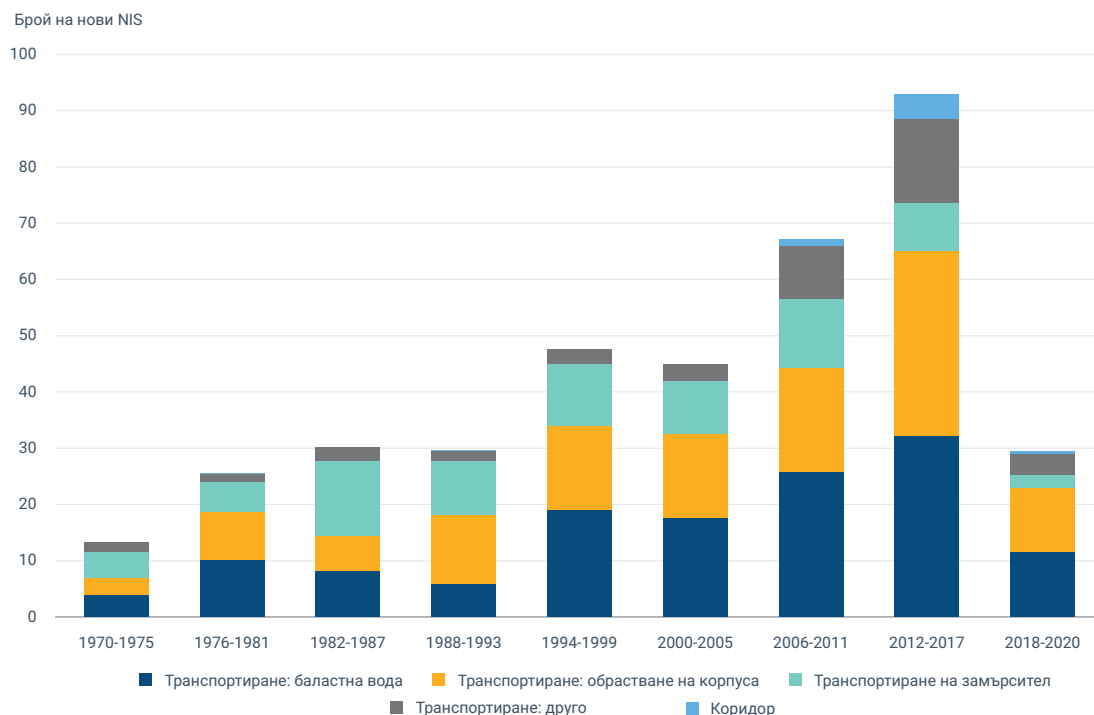
Фигура 11 Брой на новите чужди видове (NIS) в европейските регионални морета, внесени от морския транспорт, за шестгодишни цикли
