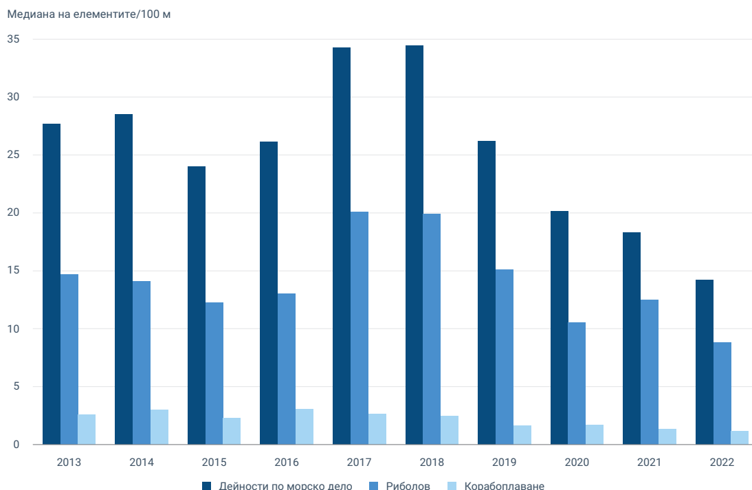
Фигура 12 Времево разпределение на отпадъците, за които е вероятно да произхождат от всички морски дейности, корабоплаване, риболов, рибни стопанства и морски култури, в европейски регионални морета
